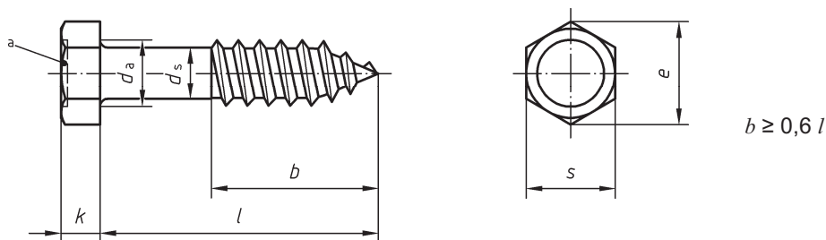
Bild 1 — Sechskant-Holzschraube
