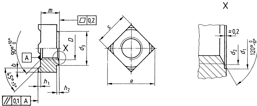
Bild 1 — Maße
