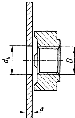
Bild 3 — Anschlussmaße (Mutter noch nicht angeschweißt)
