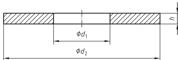
Bild 1 — Maße
